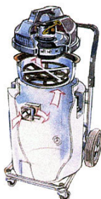
Behälter mit Filtereinsatz
