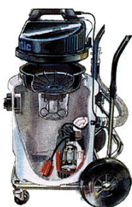
Automatische Tauchpumpe Behälter voll - Pumpe ein Behälter leer - Pumpe aus
